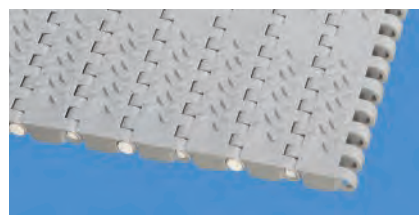
S8 | 0%开孔率 | 防滑型表面
