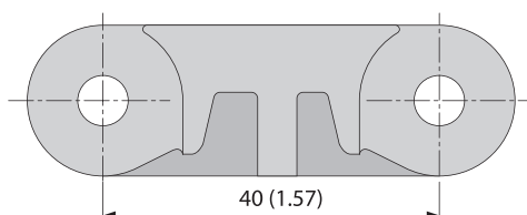
侧视图比例1:1
