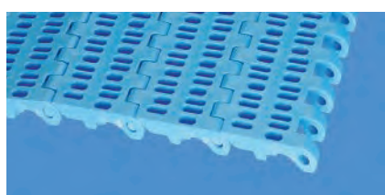
S6.1 | 23%开孔率 | 平板型表面
