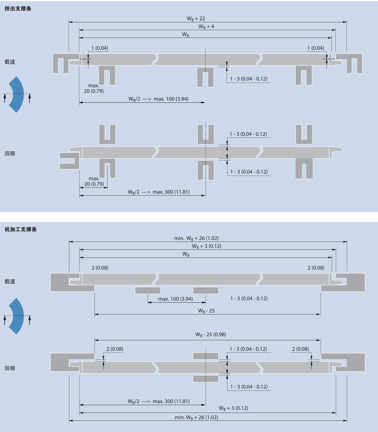
支撑条设置，S11 带钩板型盖帽
